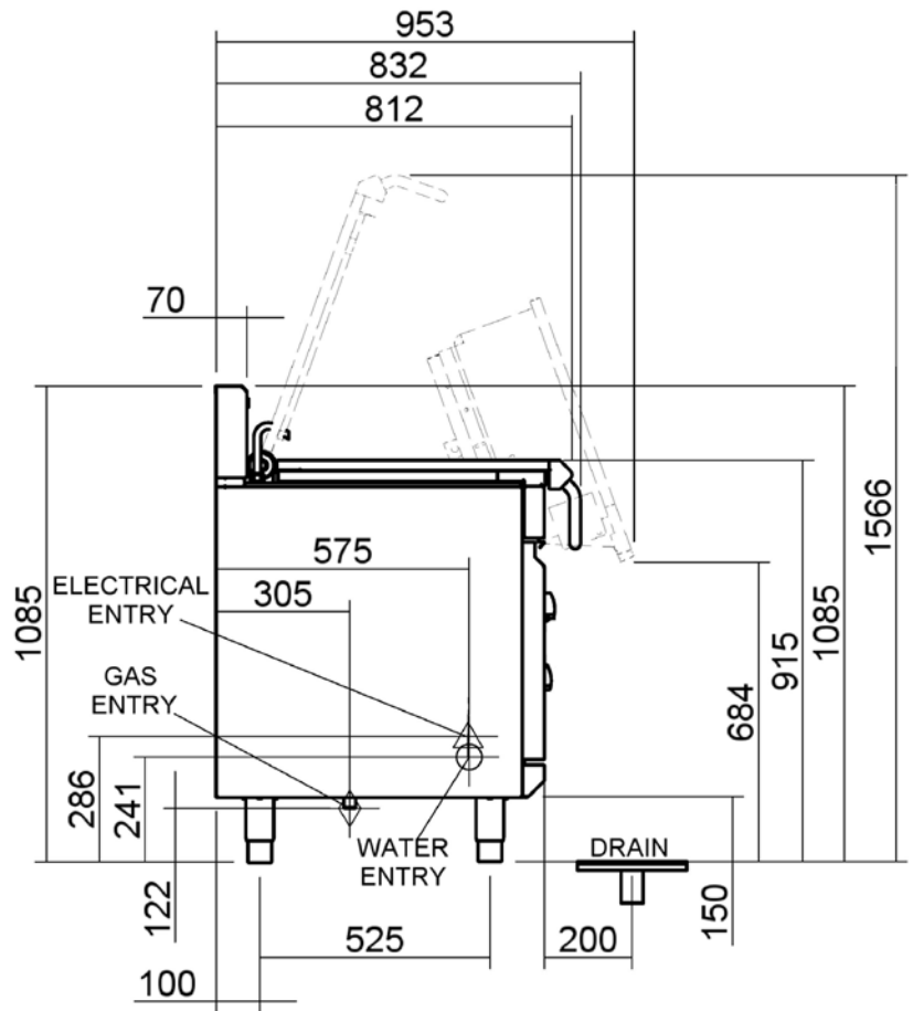
SIDE G580-8E
