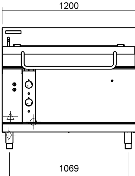
FRONT G580-12E
