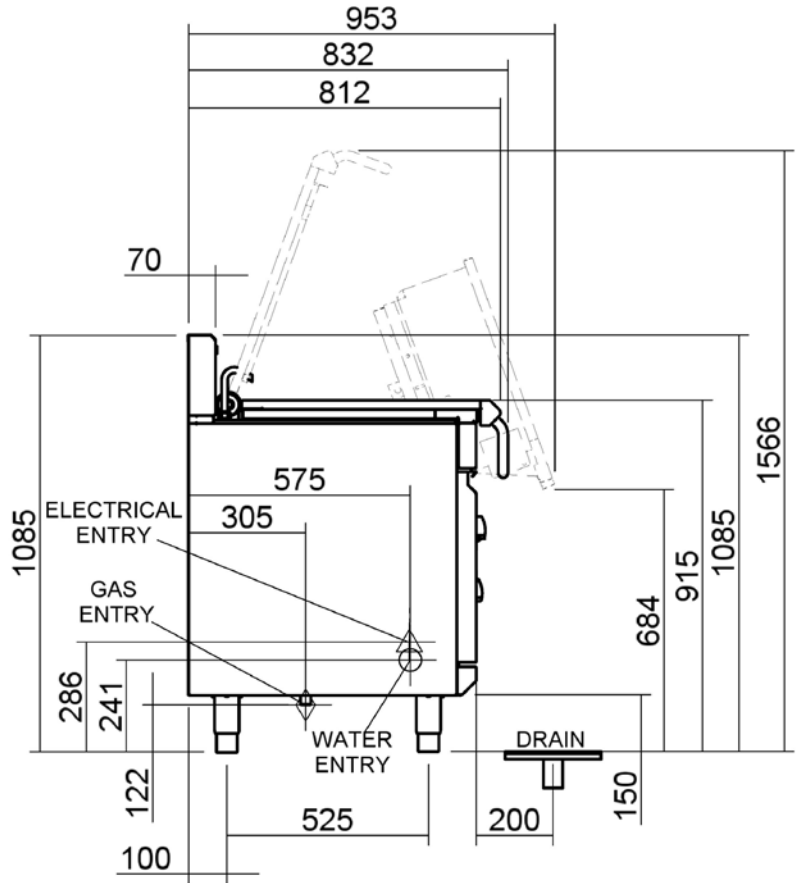
SIDE G580-12E
