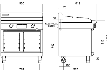
EP516-CB
