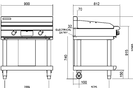
EP516-LS
